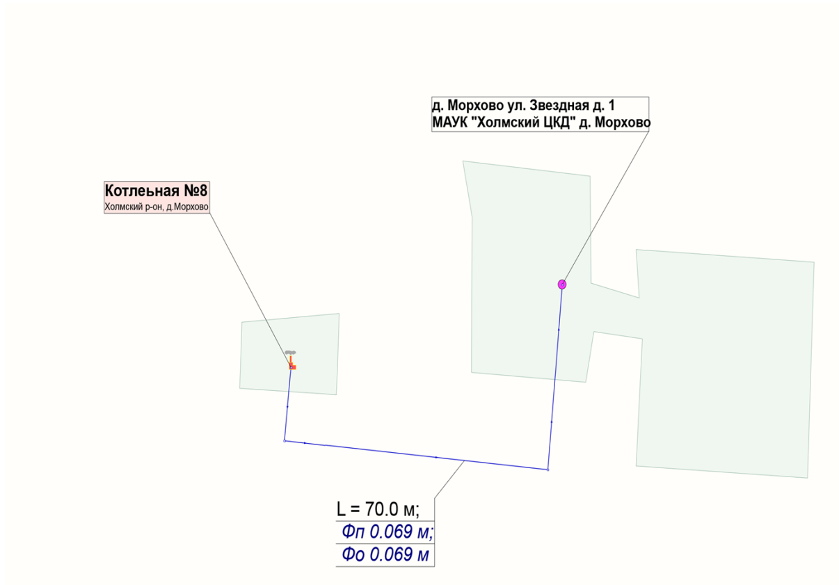
Рисунок 1.1 Схема тепловых сетей котельной №8, д. Морхово
