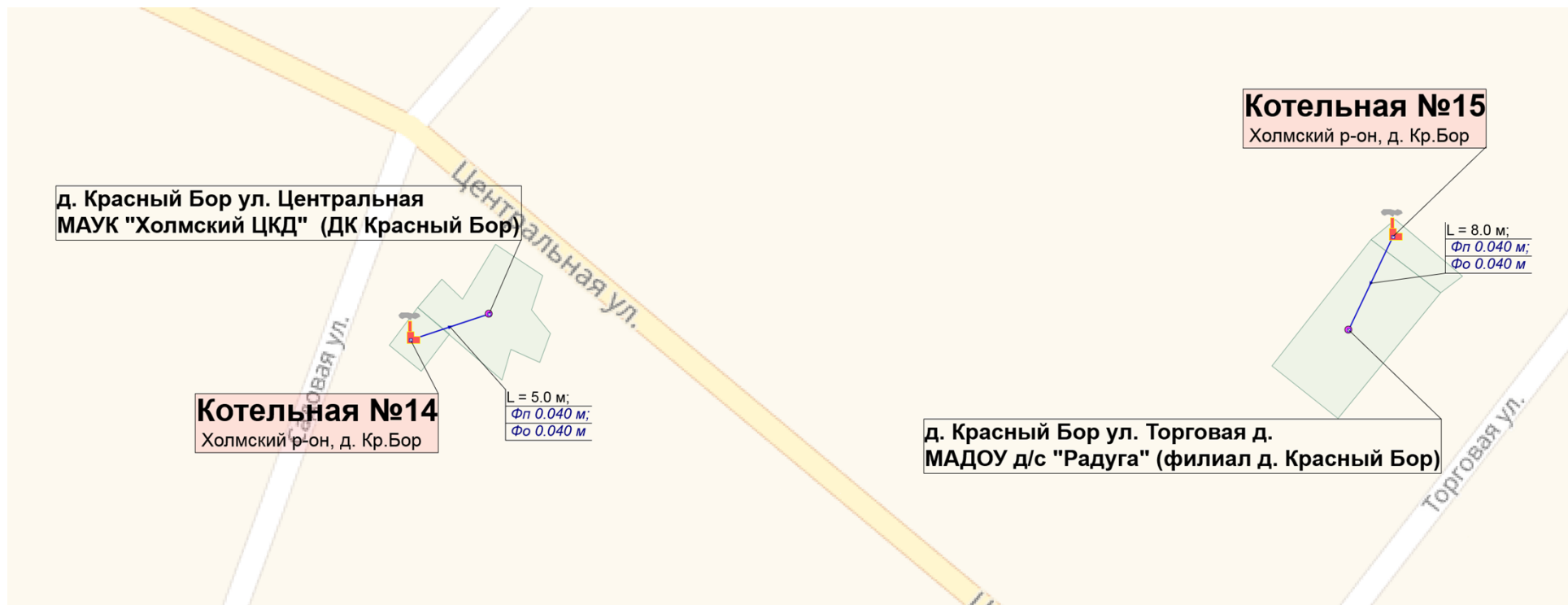
Рисунок 1.1 Схема тепловых сетей котельной №14 и №15
