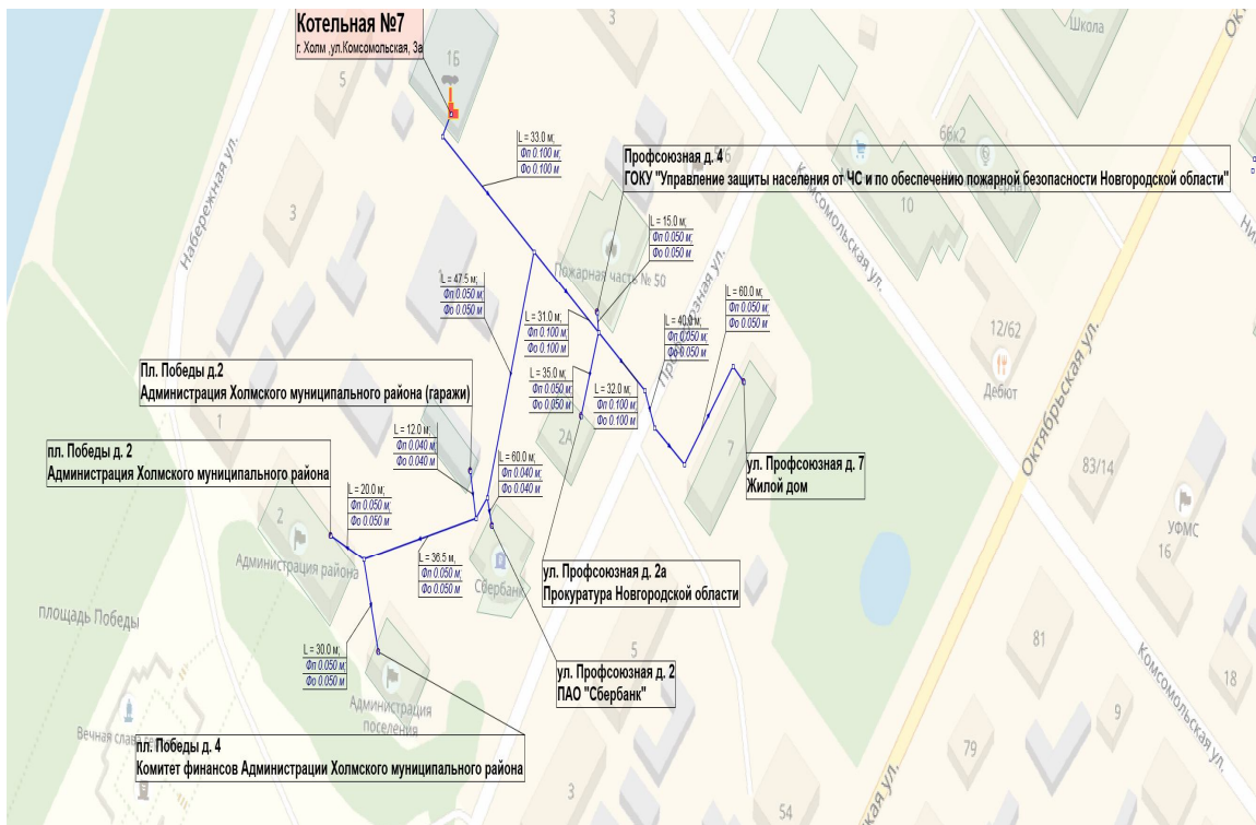
Рисунок 1.5. - Схема тепловых сетей Котельной № 7, г. Холм, ул. Комсомольская, д. 3а
