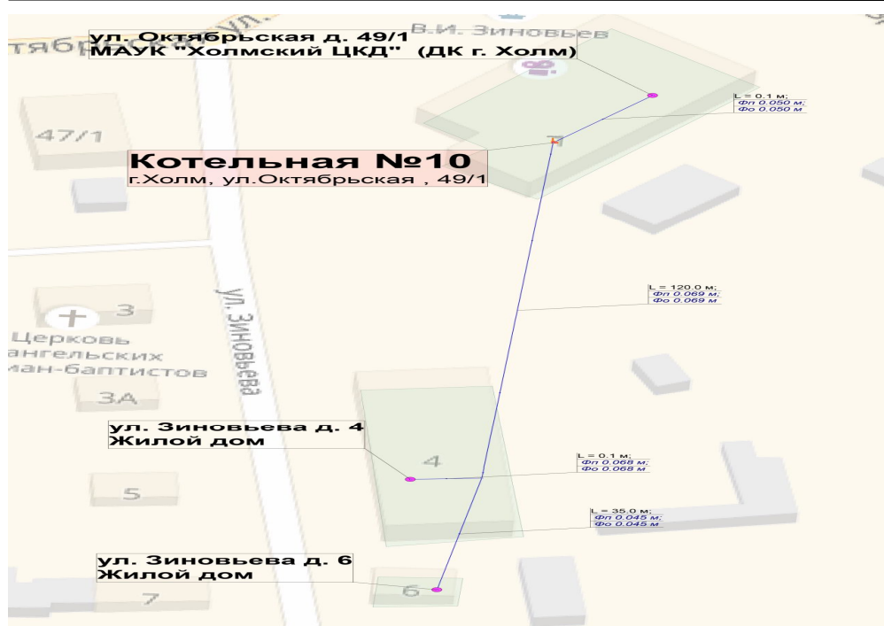
Рисунок 1.6. - Схема тепловых сетей Котельной № 10, г. Холм, ул. Октябрьская, д. 49/1
