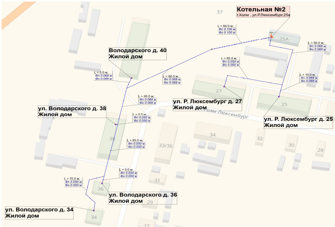
Рисунок 1.2. - Схема тепловых сетей Котельной № 2, г. Холм, ул. Р. Люксембург, д. 25а
