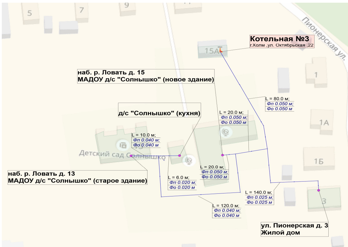
Рисунок 1.3. - Схема тепловых сетей Котельной № 3, г. Холм, ул. Октябрьская, д. 22
