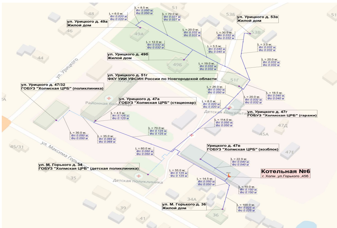
Рисунок 1.4. - Схема тепловых сетей Котельной № 6, г. Холм, ул. Горького, д. 456
