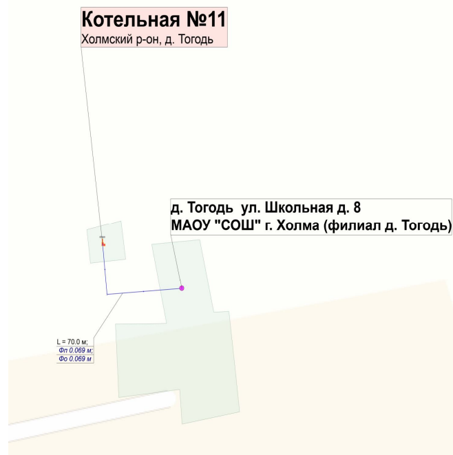
Рисунок 1.1 Схема тепловых сетей котельной №11
