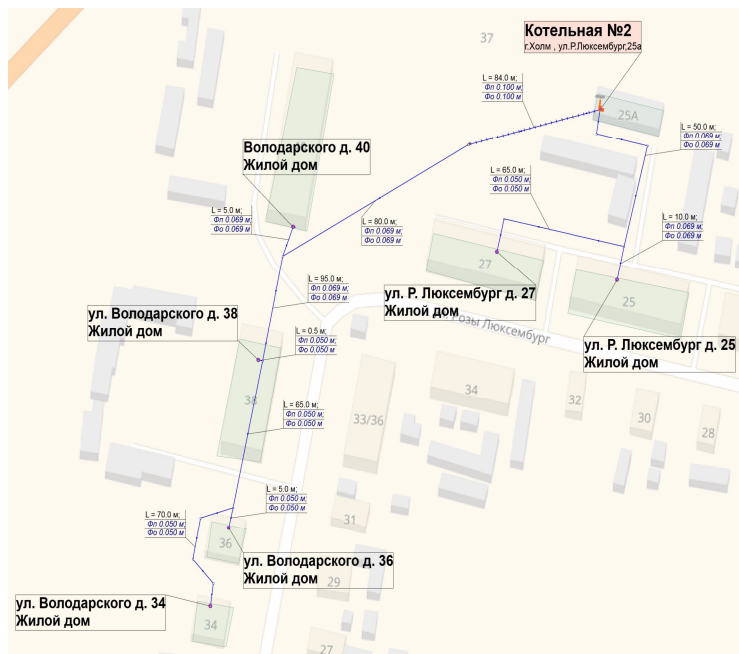
Рисунок 1.2. - Схема тепловых сетей Котельной № 2, г. Холм, ул. Р.Люксембург, д. 25а
