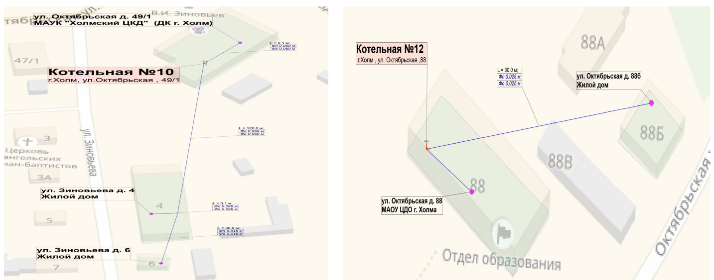
Рисунок 1.7. - Схема тепловых сетей Котельной №12, г. Холм, ул. Октябрьская, 88
