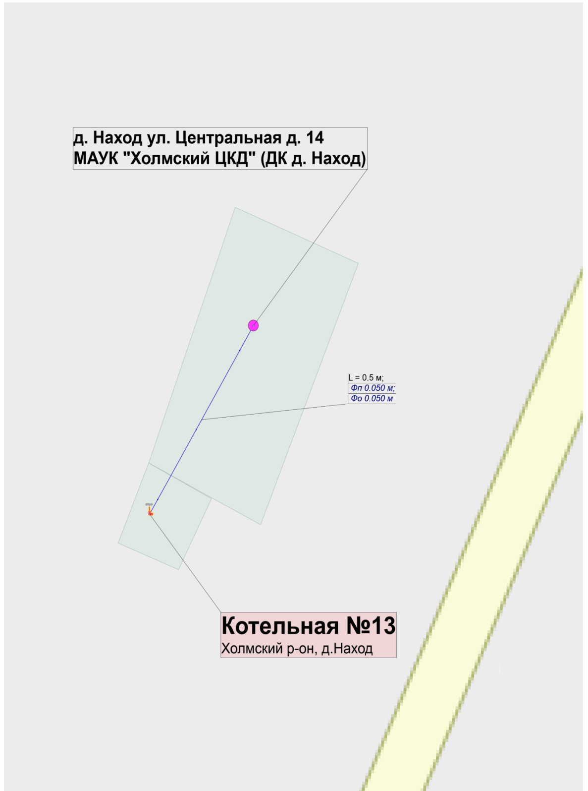
Рисунок 1.2 Схема тепловых сетей котельной №13
