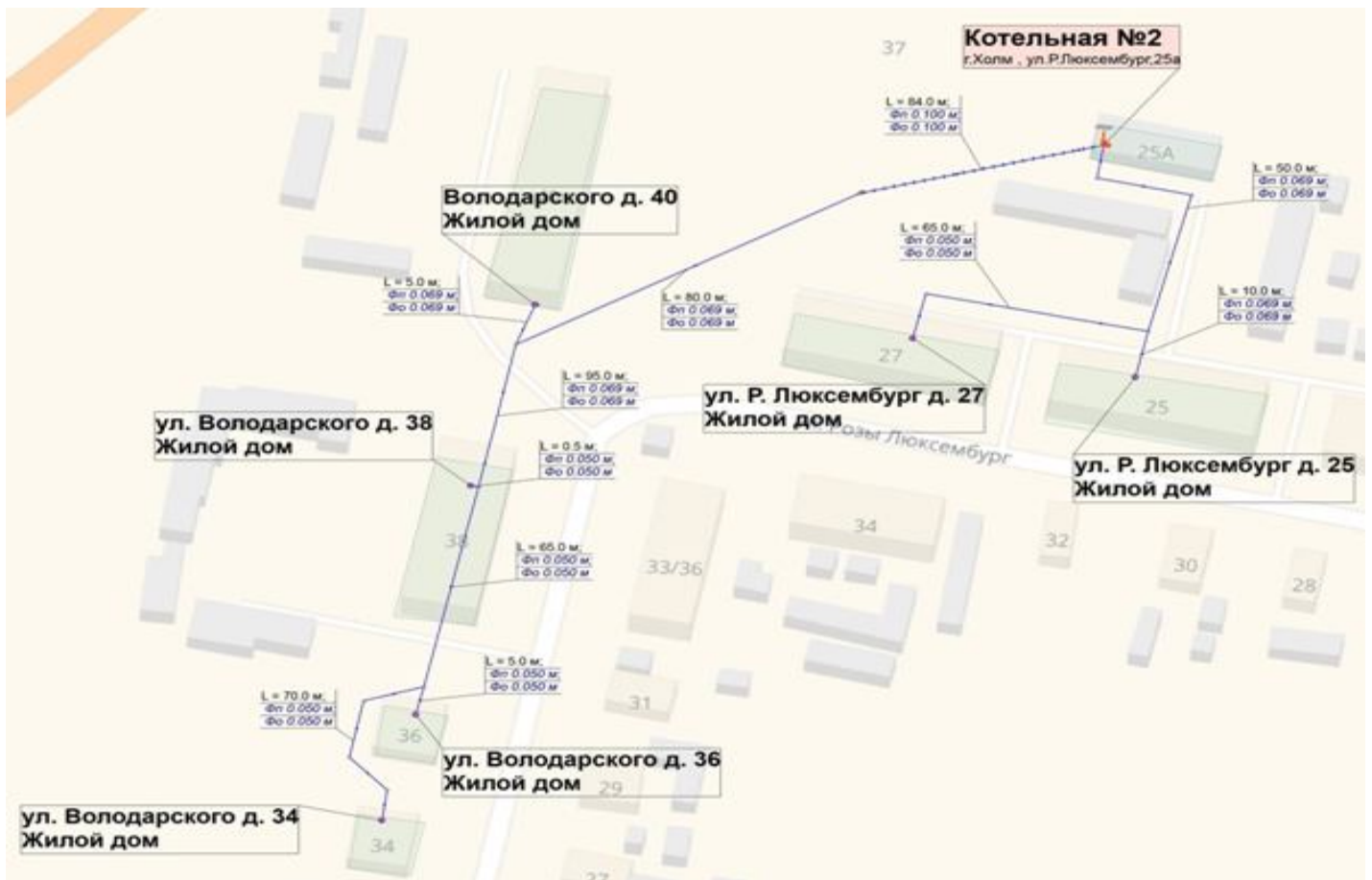
1.3.2.2 Схема тепловой сети от источника тепловой энергии Котельная №2
