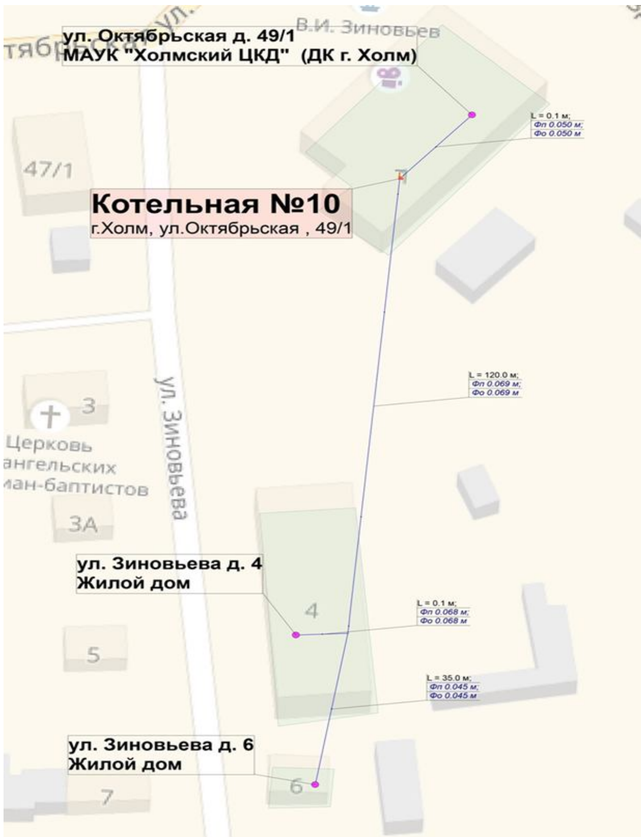
1.3.2.6 Схема тепловой сети от источника тепловой энергии Котельная № 10
