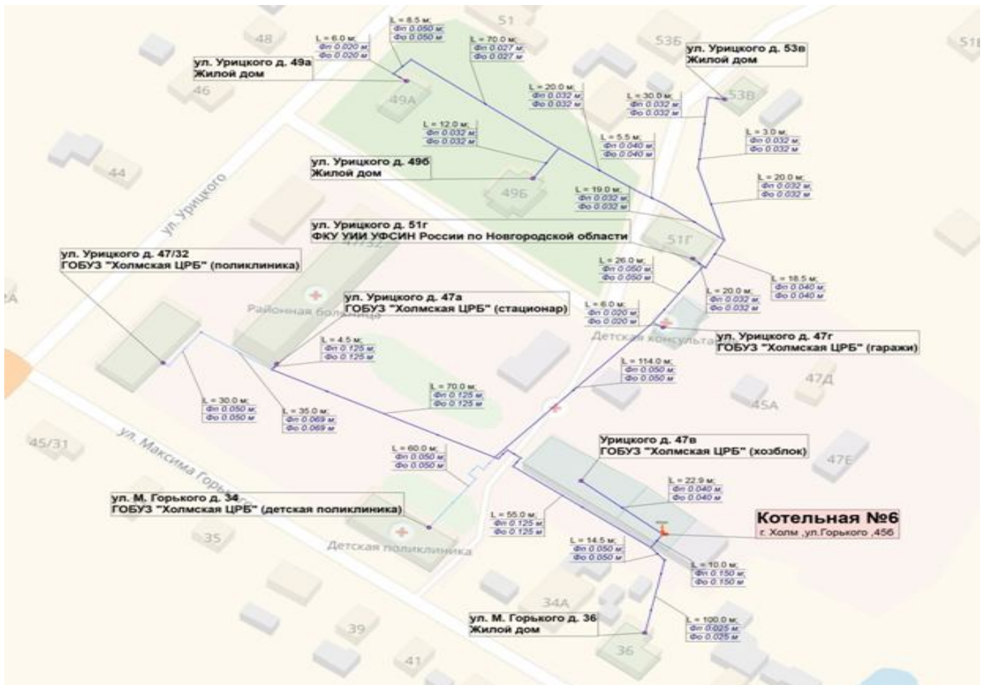
1.3.2.4 Схема тепловой сети от источника тепловой энергии Котельная №6
